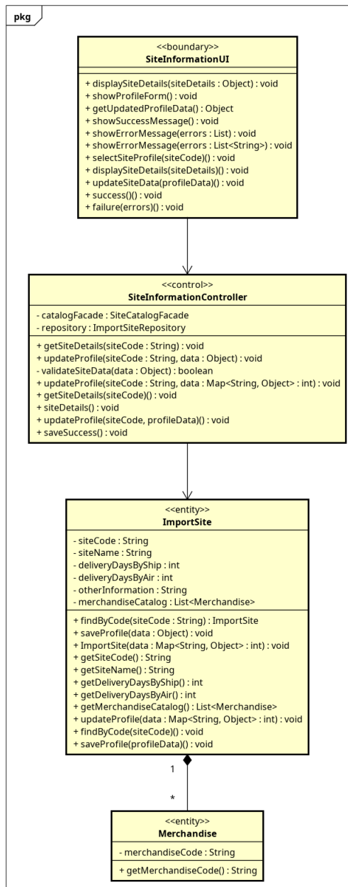
Hình 2.3: Class diagram mức phân tích UC002 - ManageSiteInformation
