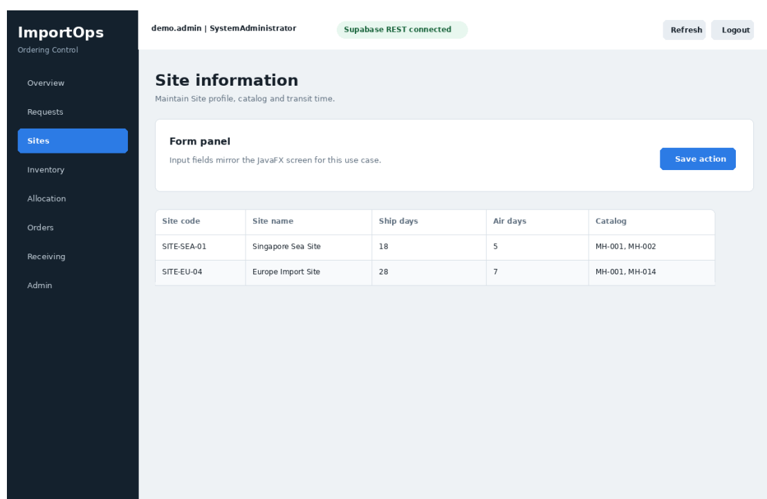
Hình 3.2: Giao diện quản lý hồ sơ Site
