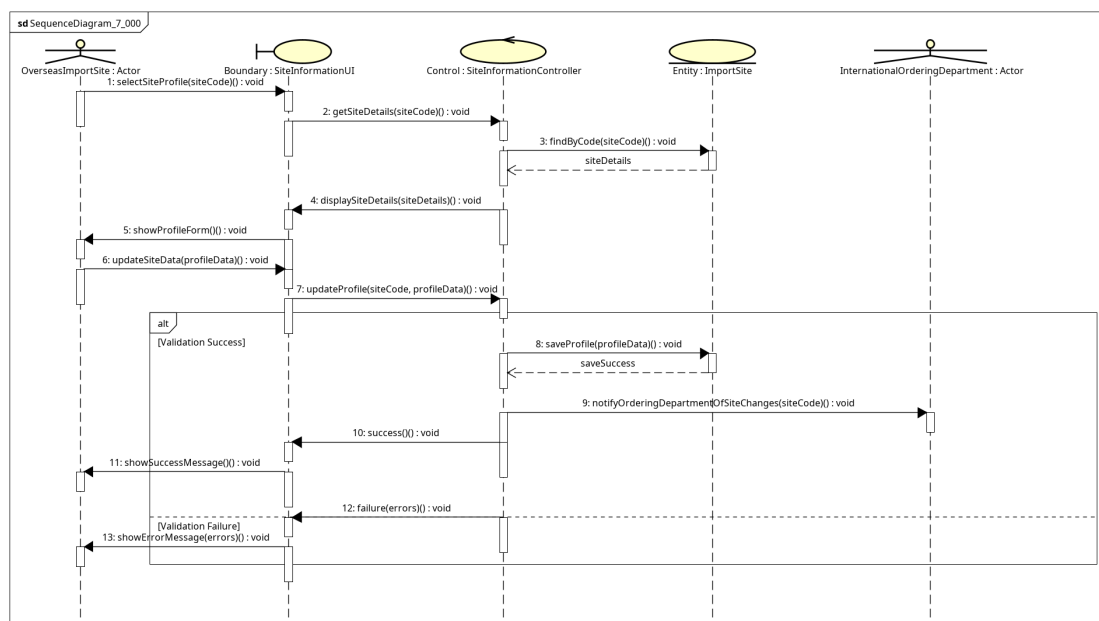
Hình 2.1: Sequence diagram mức phân tích UC002 - ManageSiteInformation
