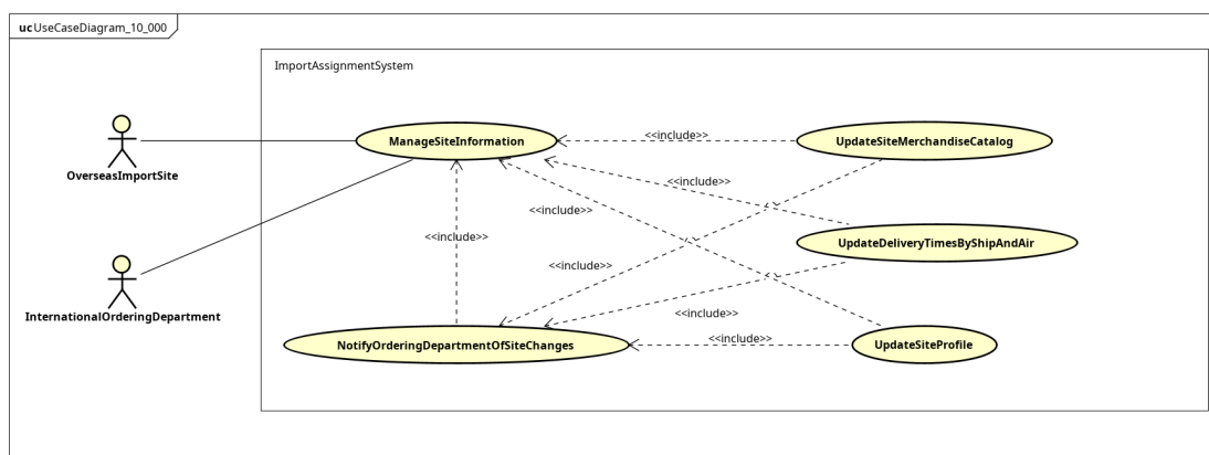
Hình 1.1: Use case phân rã UC002 - ManageSiteInformation
