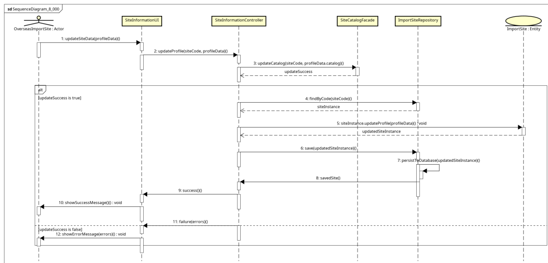
Hình 4.1: Sequence diagram mức thiết kế UC002 - ManageSiteInformation
