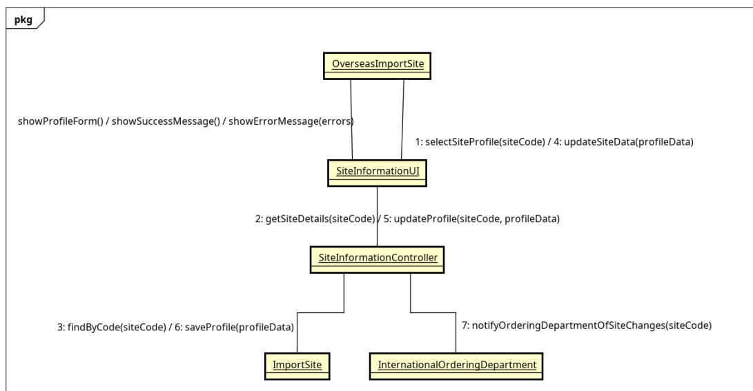
Hình 2.2: Communication diagram mức phân tích UC002 - ManageSiteInformation
